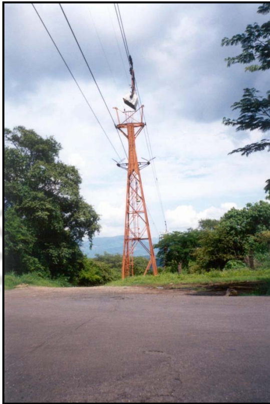
Teleférico que transporta el mineral de la mina El Encino a la planta peletizadora de estación alzada, Mpio. de Cuauhtémoc, Col.
